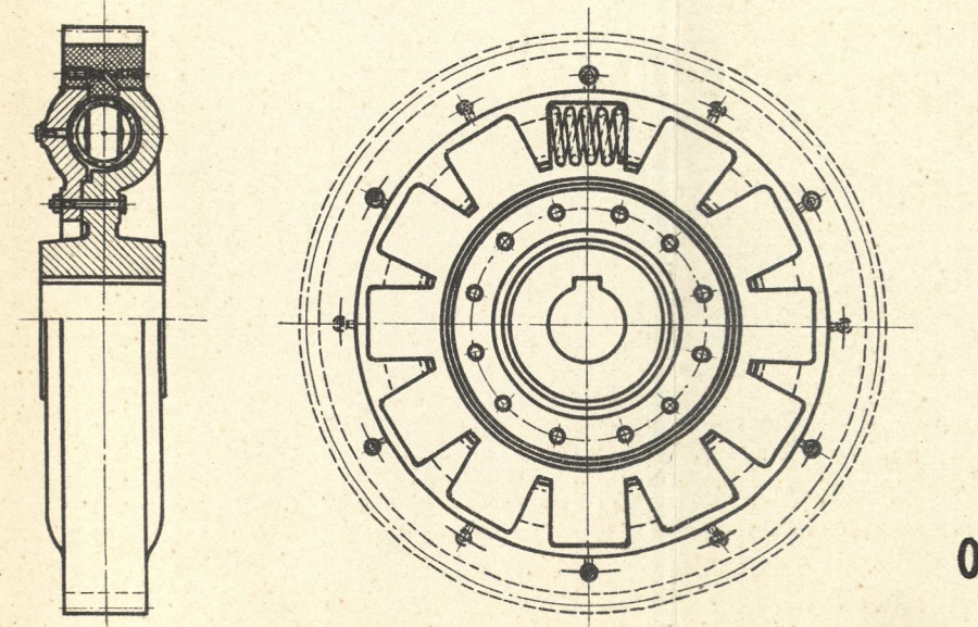
VEEREND TANDWIEL.
