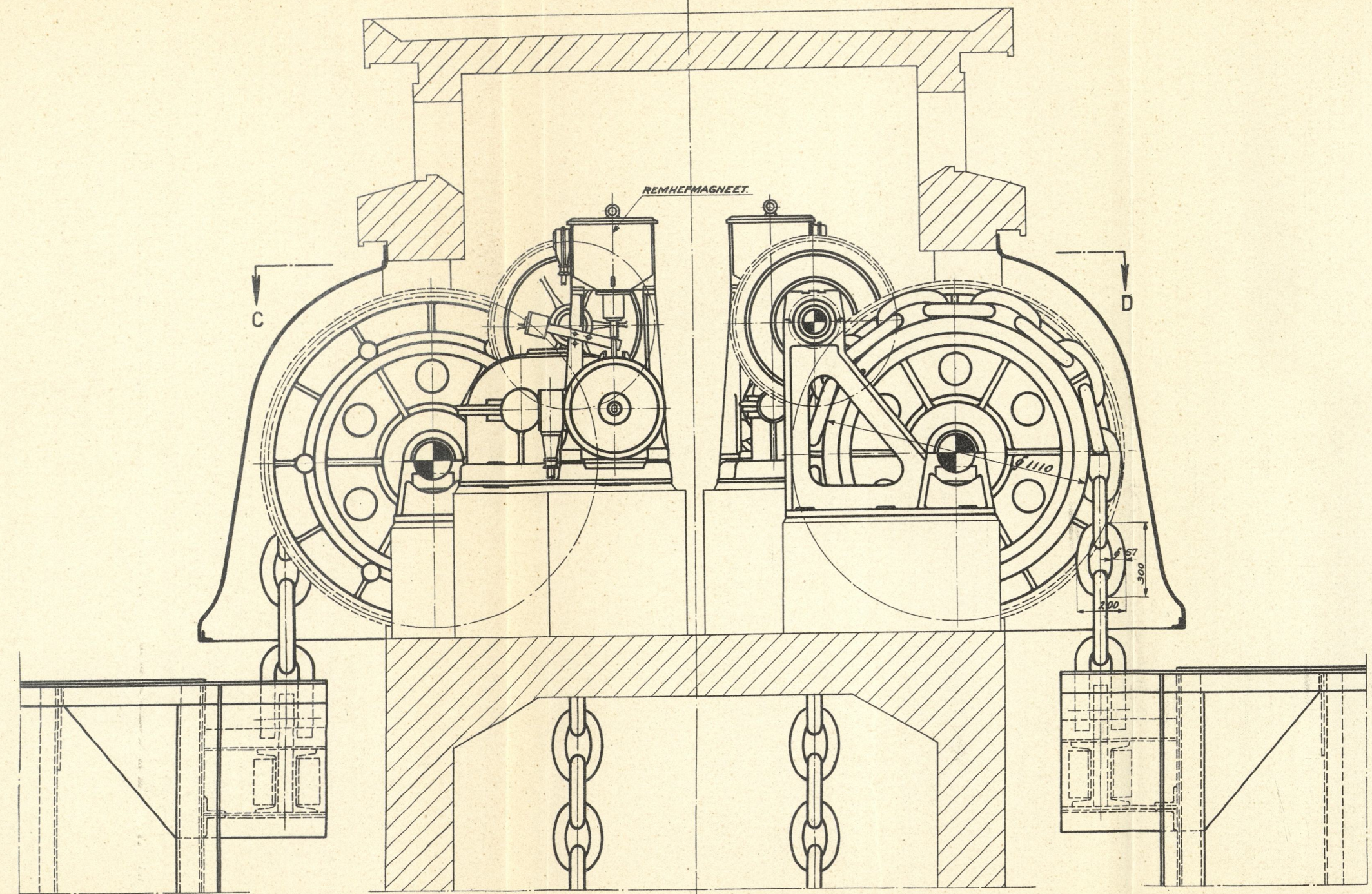
DOORSNEDE A-B.
