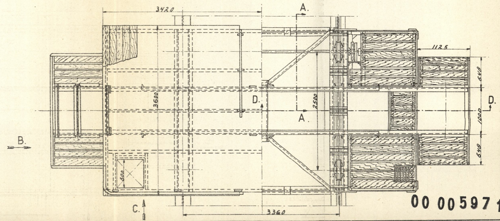
BOVENAANZICHT OP DAK.
