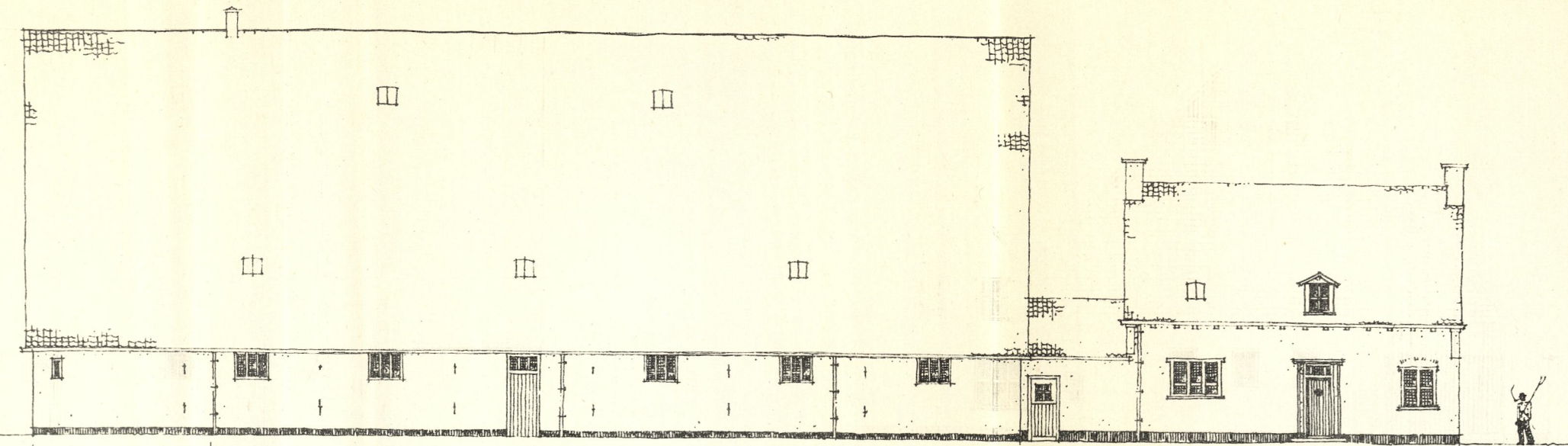
linkerzijgevel.
