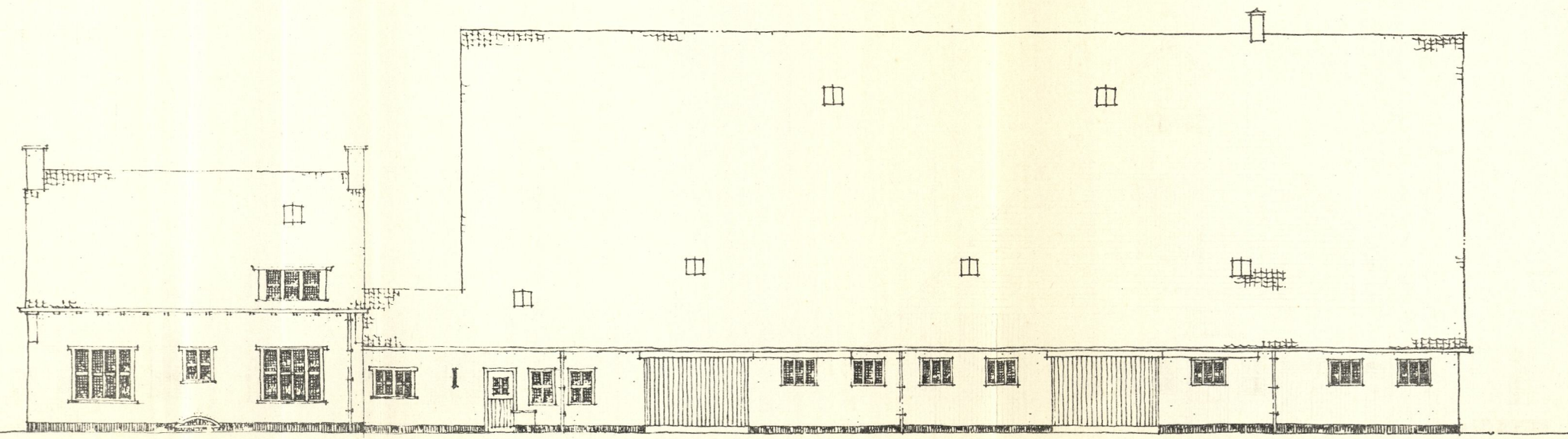
rechterzijgevel.
