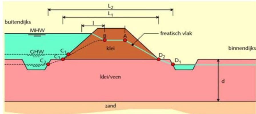
Figuur 4.1 Schematisatie freatisch vlak voor STBI-1, kleilig kernmateriaal
