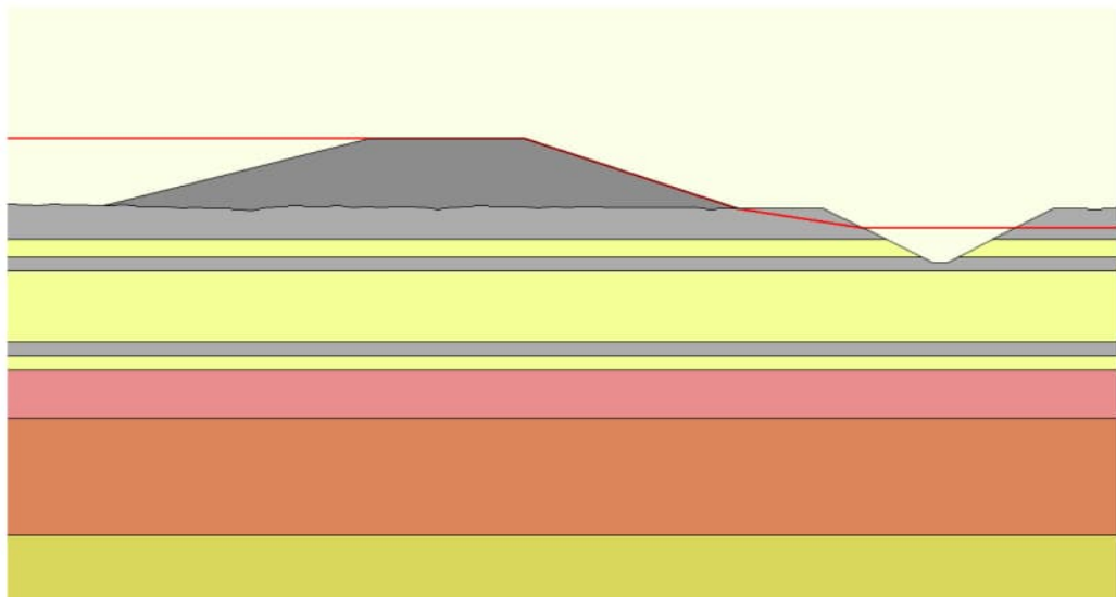
Figuur 4.3 STBI-1 hoge kade overlaatsectie, kleiig kernmateriaal
