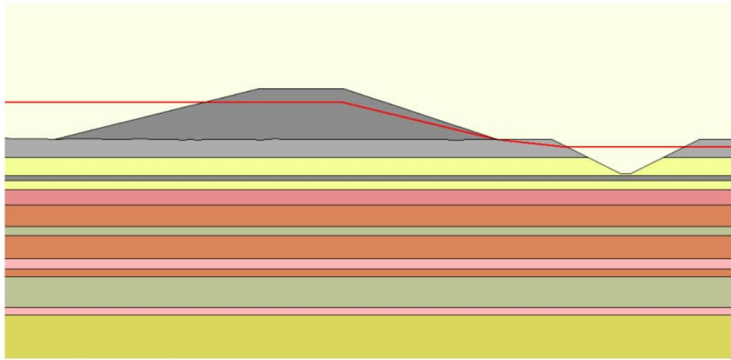
Figuur 4.2 STBI-1 hoge kade geen overlaatsectie, kleiig kernmateriaal
