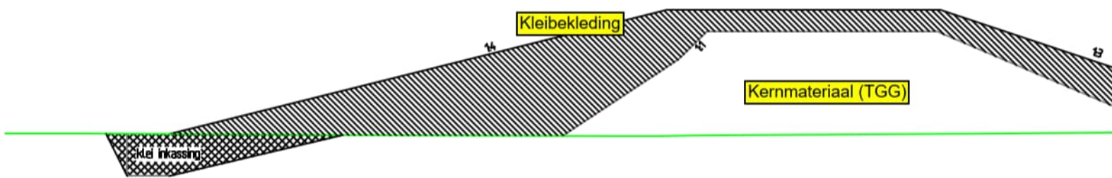
PRINCIPEPROFIEL KLEIBEKLEDING EN KLEI INKASSING HOGE KAD
