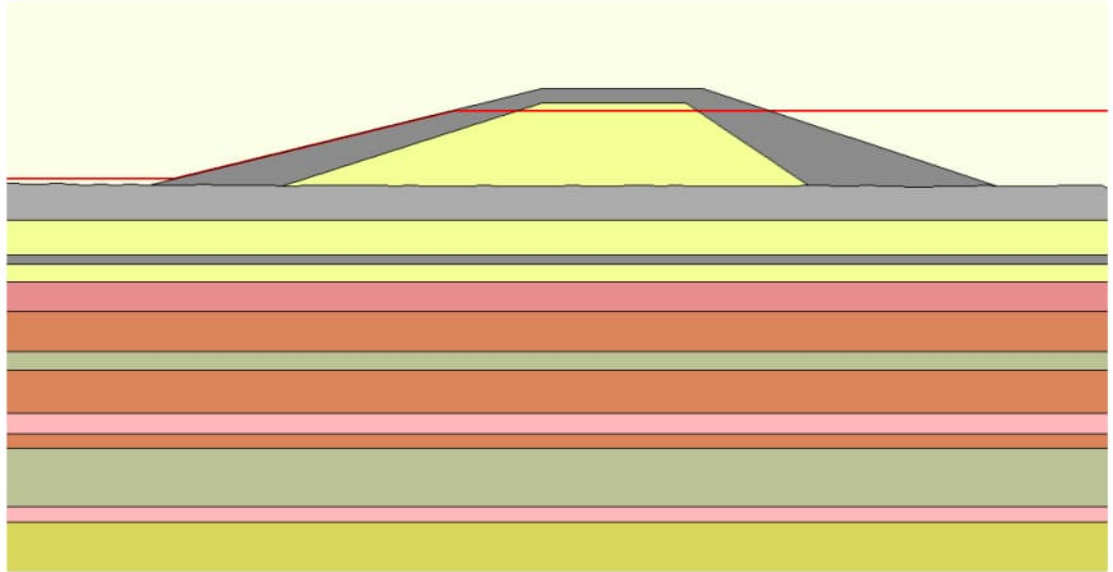
Figuur 4.10 STBU-2 (geen overlaat, kleiig of zandig kernmateriaal)
