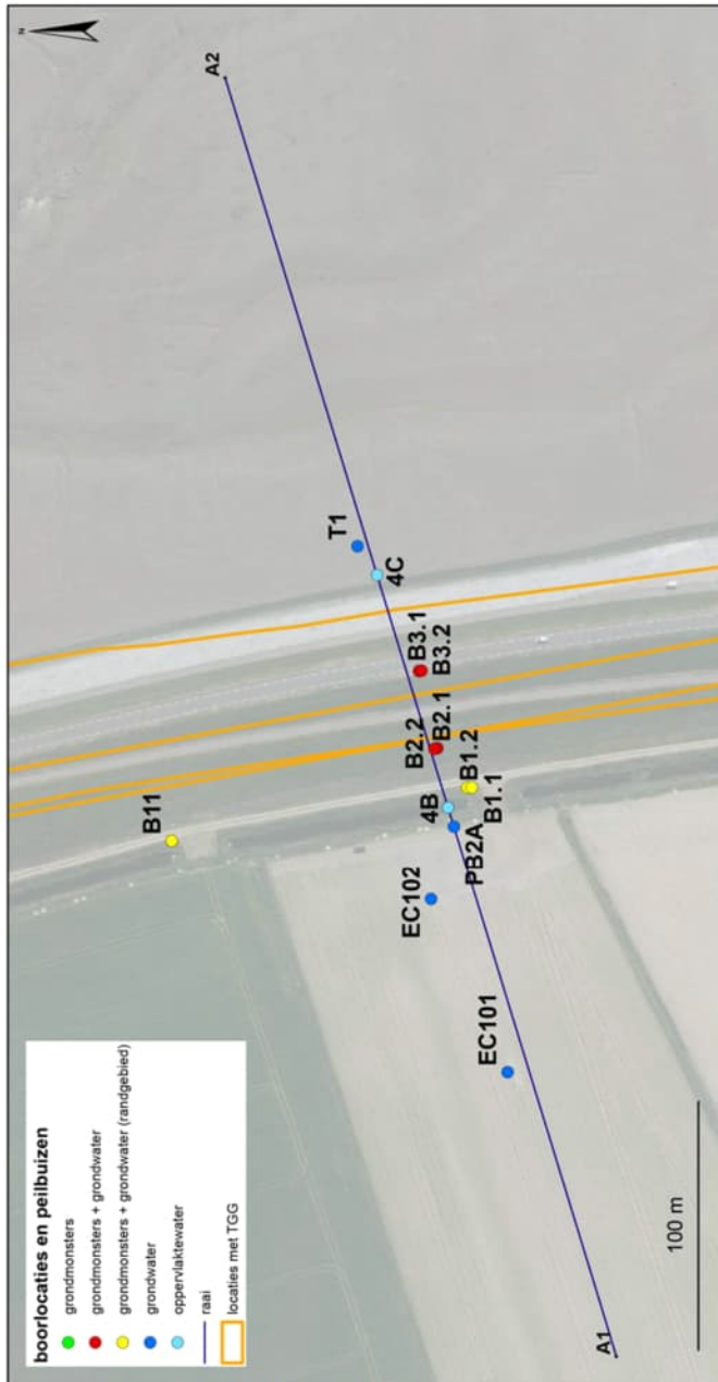
Figuur 2.6 Detail informatie van Meetraai A1-A2
