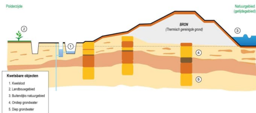
Figuur 2.3 Schematische weergave van de zeedijk, aanwezigheid van thermisch gereinigde grond (TGG), kwetsbare objecten en bodemopbouw: geel = zand, rood-bruin = klei en donkerbruin = veen. De bodemopbouw ter plaatse van de intensere kleuren is afgeleid op basis van uitgevoerde boringen
