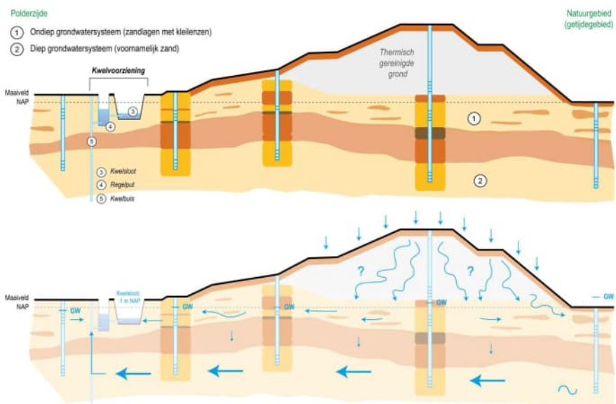
Figuur 3.8 Conceptueel diagram van de (grond)waterstroming. GW = grondwaterstroming, Geel = zand, rood-bruin = klei en donkerbruin = veen. Sinuslijntje stelt invloed van getij voor, NAP = Normaal Amsterdams Peil
