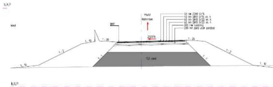
Figuur 4.23 Constructieopbouw knoppunt Princeville
