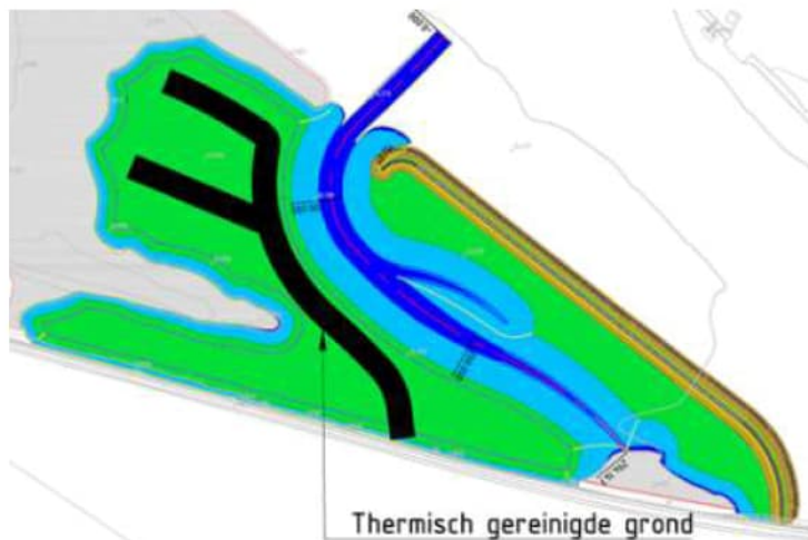
Figuur 4.18 Toepassing TGG op locatie Grote Zaag (bron: tekening door Martens en Van Oord, 28 mei 2016, behorende bij BKKBBK-melding)
