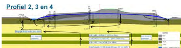
Figuur 2.1: principeprofiel grondwaterstroming
