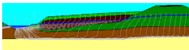
Figuur 2.2: gemodelleerd profiel grondwaterstroming
