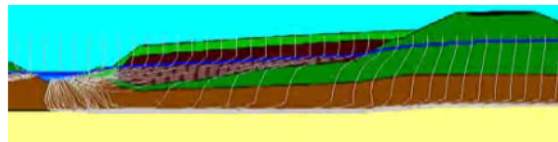
Figuur 2.2: gemodelleerd profiel grondwaterstroming
