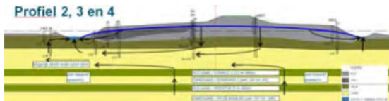
Figuur 2.1: principeprofiel grondwaterstroming
