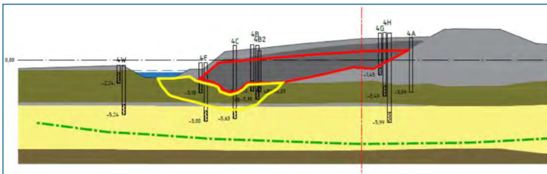
Figuur 1.1: Principeschets bromideverontreiniging
