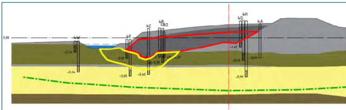
Figuur 2.4: Principeschets bromideverontreiniging
