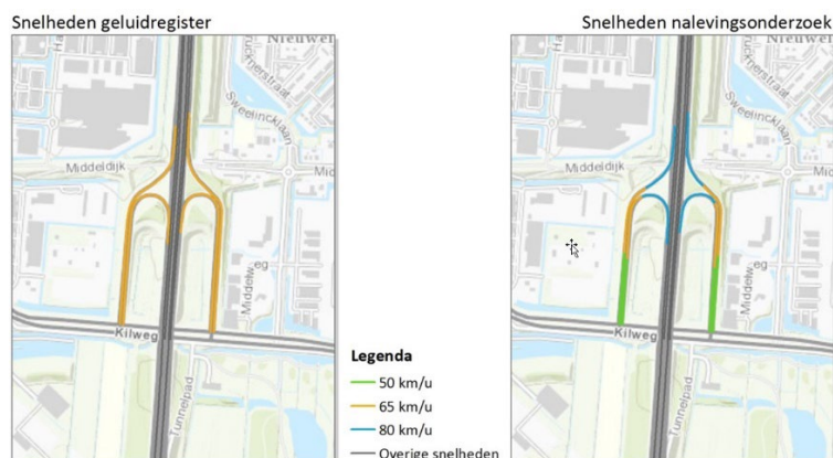
Afbeelding 3-4 Aanpassing representatieve snelheden op toe- en afritten
