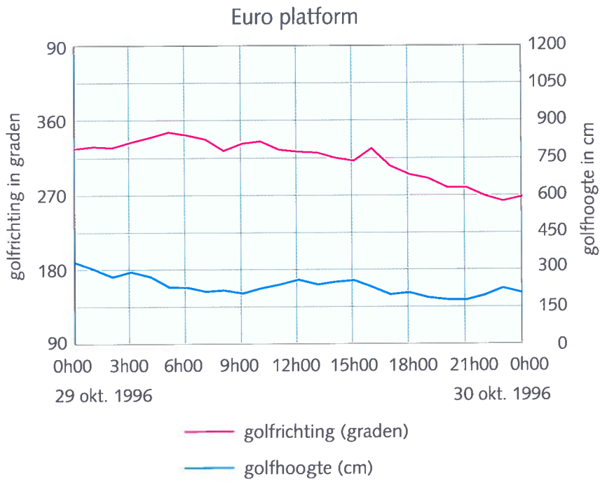
Figuur 6 Verloop Golfhoogten en -richtingen Euro platform
