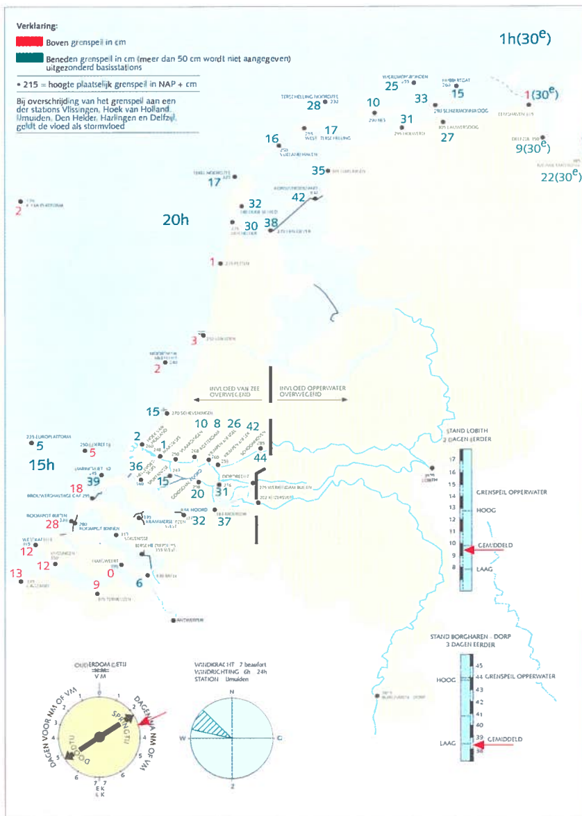
Figuur 5 Opgetreden hoogwaterstanden van 29 oktober 2 e hoogwater t.o.v. plaatselijke grenspeerl.
