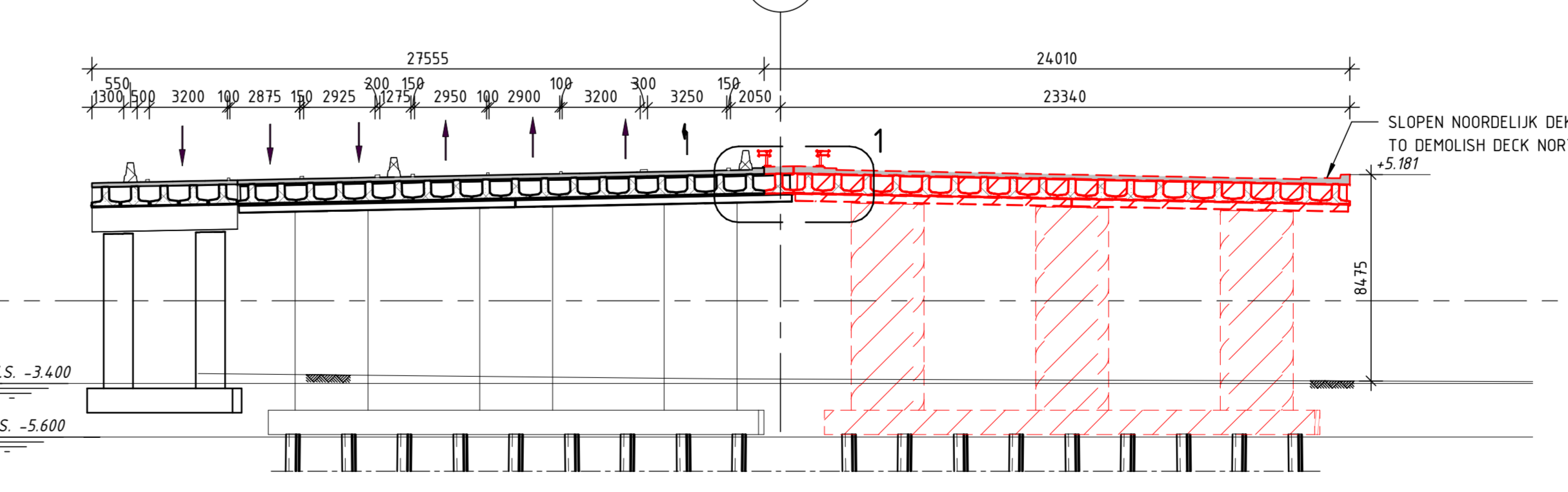
DOORSNEDE B-B / SECTION B-B schaal: 1: 200
