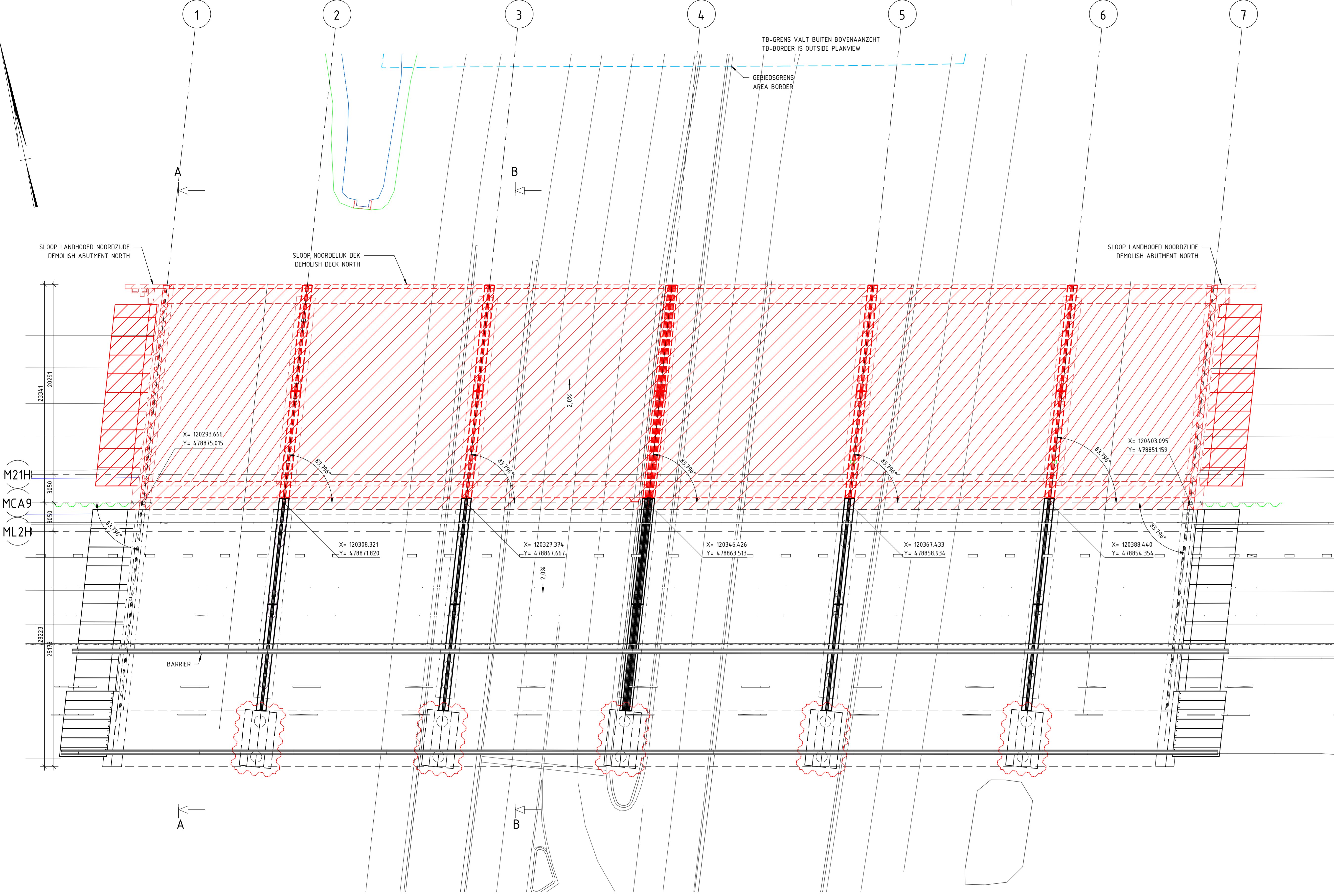
BOVENAANZICHT FASE 4 SLOOP / PLANVIEW PHASE 4 TO DEMOLISH schaal: 1: 200
