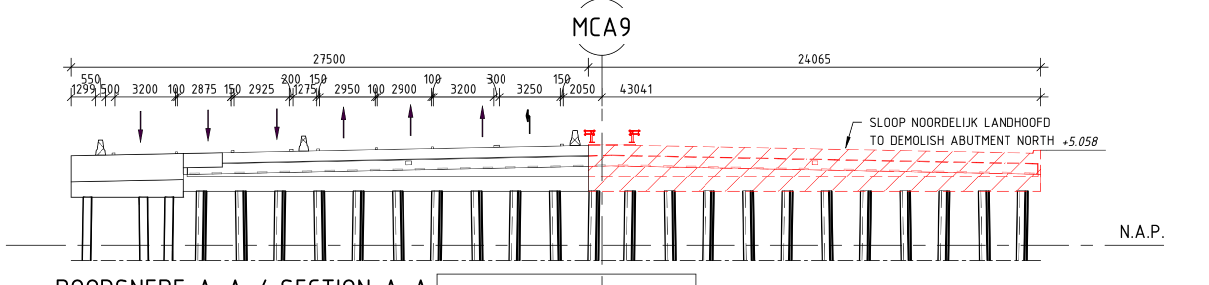
DOORSNEDE A-A / SECTION A-A DEK NIET GETEKEND / DECK NOT DRAWN schaal: 1: 200
