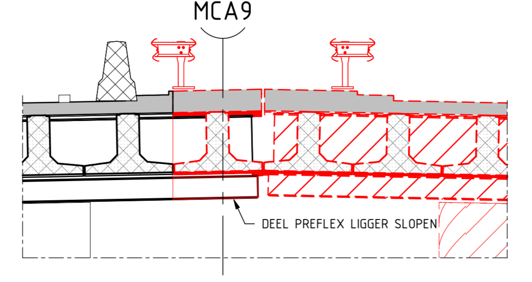
DETAIL 1 schaal: 1: 50
