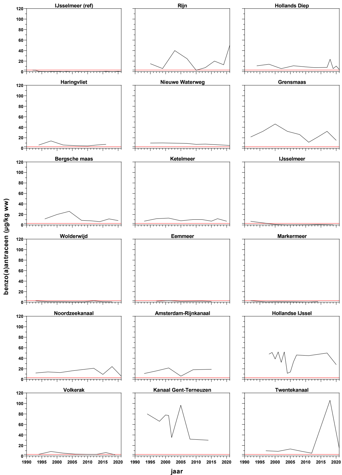
Figuur 48 KRW toetswaarden 1992 tot en met 2021 van benzo(a)antracene uitgedrukt in natgewicht standaard schelpdier gemeten in de actieve biologische monitoring van schelpdieren in zoetwater. De rode lijn geeft de EQS biota aan.
