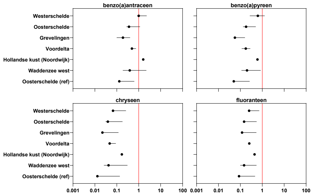
Figuur 17 Meest recente meetwaarde (stippen; jaar 2020, alleen Hollandse kust (Noordwijk) 2017) en de range van gemeten waarden sinds 1992, genormaliseerd ten opzichte van de EQS biota (=1, rode verticale lijn) voor de PAK's gemeten in blauwe mossel (ABM).
