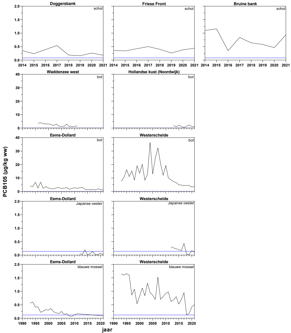
Figuur 55 Gehalten van PCB105 uitgedrukt op basis van natgewicht gemeten in vislevens (schol en bot) en in schelpdiervlees (Japanse oester en blauwe mossel) uit de passieve biotamonitoring in zoutwater voor OSPAR. Periode 1991 tot en met 2021. Blauwe lijn is de BAC.
