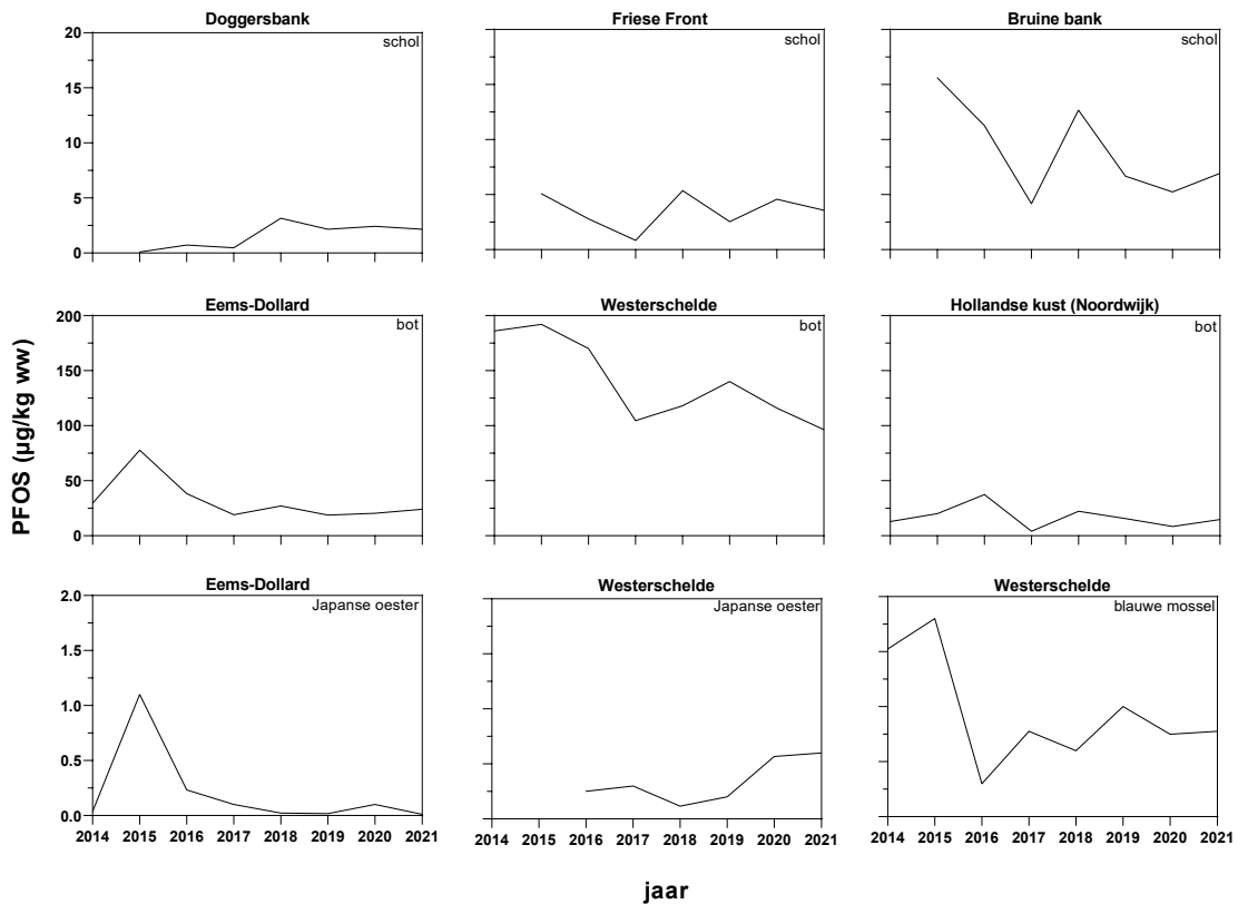
Figuur 35 Gehalten van PFOS uitgedrukt in µg/kg op basis van natgewicht gemeten in de lever van bot en schol en schelpdiervlees van blauwe mossel en Japanse oester in zoutwater. Periode 2014-2021.
