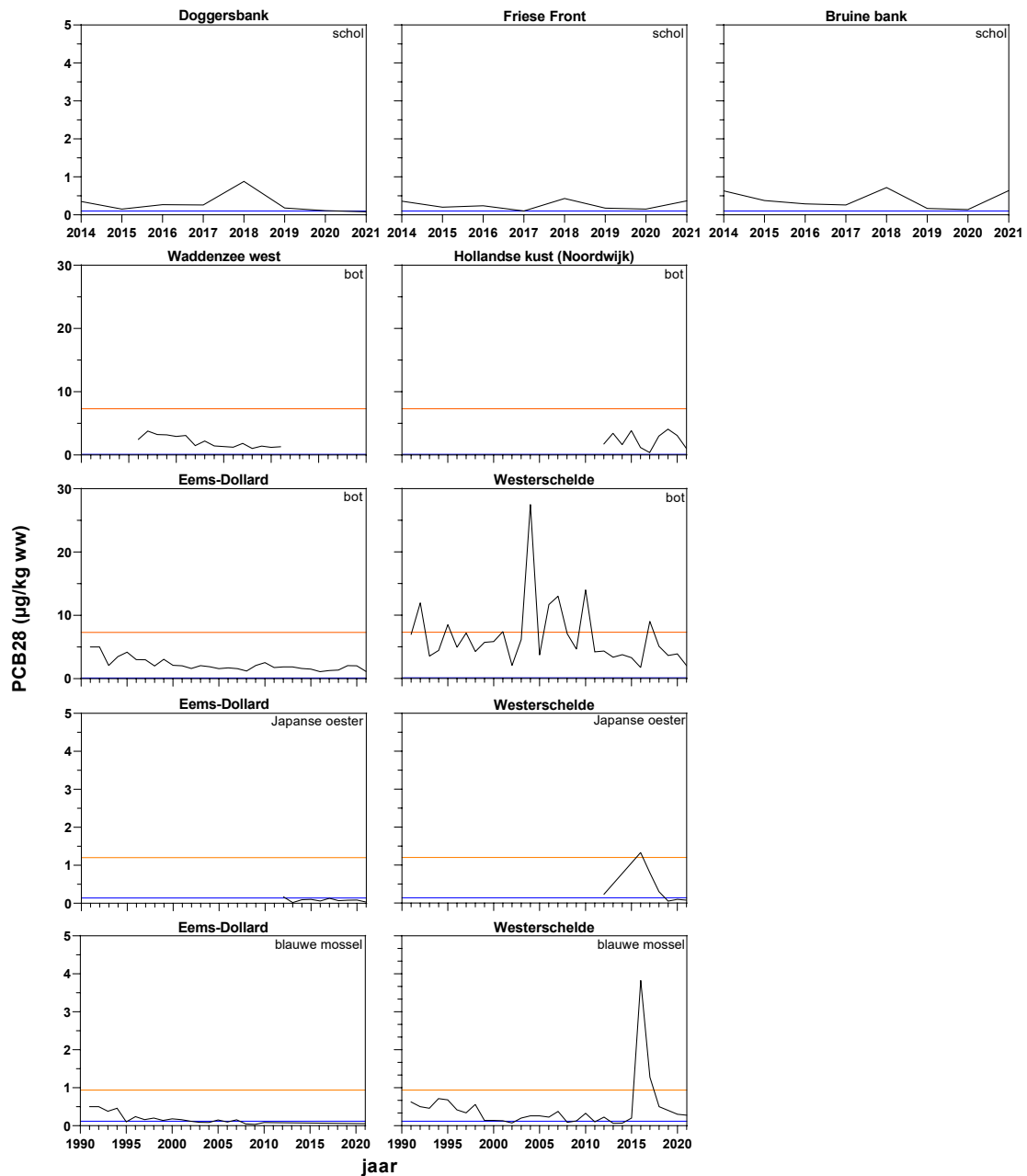
Figuur 52 Gehalten van PCB28 uitgedrukt op basis van natgewicht gemeten in vislevers (schol en bot) en in schelpdier vlees (Japanse oester en blauwe mossel) uit de passieve biotamonitoring in zoutwater voor OSPAR. Periode 1991 tot en met 2021. Blauwe lijn is de BAC en de oranje lijn is de EAC/MPC/FEQG.
