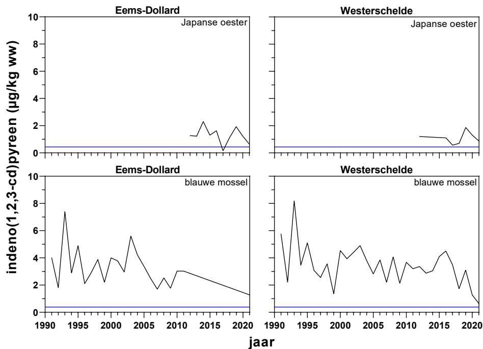
Figuur 46 Gehalten van indeno(1,2,3-cd)pyreen uitgedrukt op basis van natgewicht gemeten in schelpdieren (blauwe mossel en Japanse oester) voor OSPAR. Periode 1991 tot en met 2021. Blauwe lijn is de BAC.
