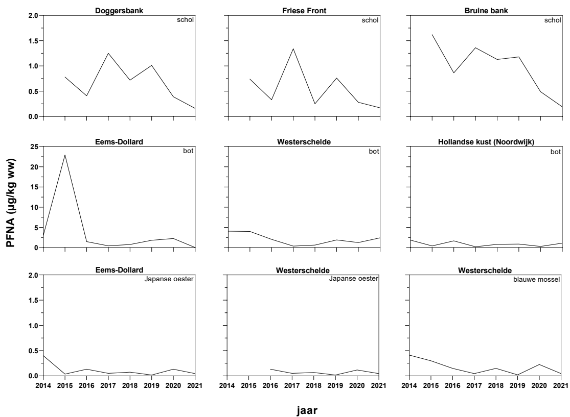
Figuur 37 Gehalten van PFNA uitgedrukt op basis van natgewicht gemeten in de levers van bot en schol en schelpdier vlees van blauwe mossel en Japanse oester uit de passieve biologische monitoring in zoutwater. Periode 2014-2021.
