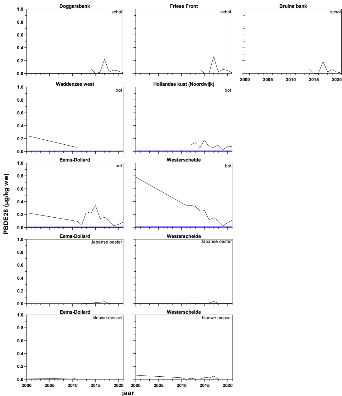
Figuur 61 Gehalten van PBDE28 uitgedrukt op basis van natgewicht gemeten in vislevers (schol en bot) en in schelpdiervlees (Japanse oester en blaauwe mossel) uit de passieve biotamonitoring in zoutwater voor OSPAR. Periode 2000 tot en met 2021. Blauwe lijn is de BAC.
