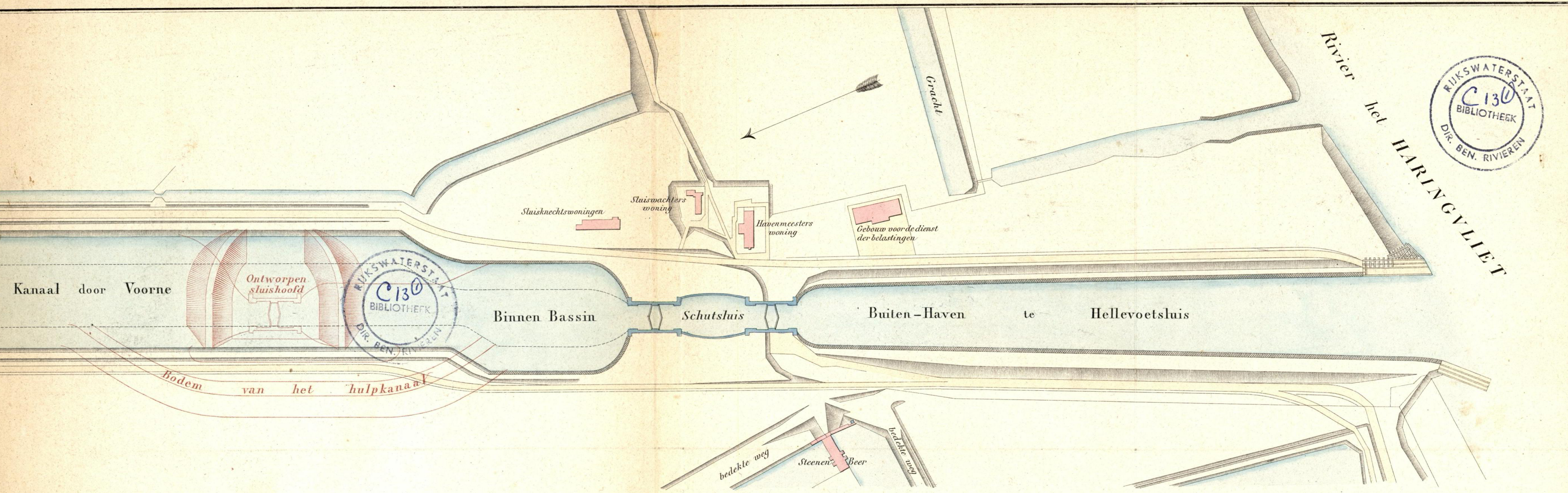
Kaart van de beide Schutsluizen in het kanaal door Voorne, waarop in roode lijnen is aangegeven, een ontwerp tot het bouwen van een derde sluishoofd, bij ieder dier sluizen.
