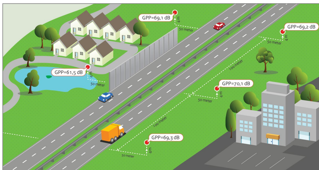
Afbeelding 2-1 Schematische weergave referentiepunten
