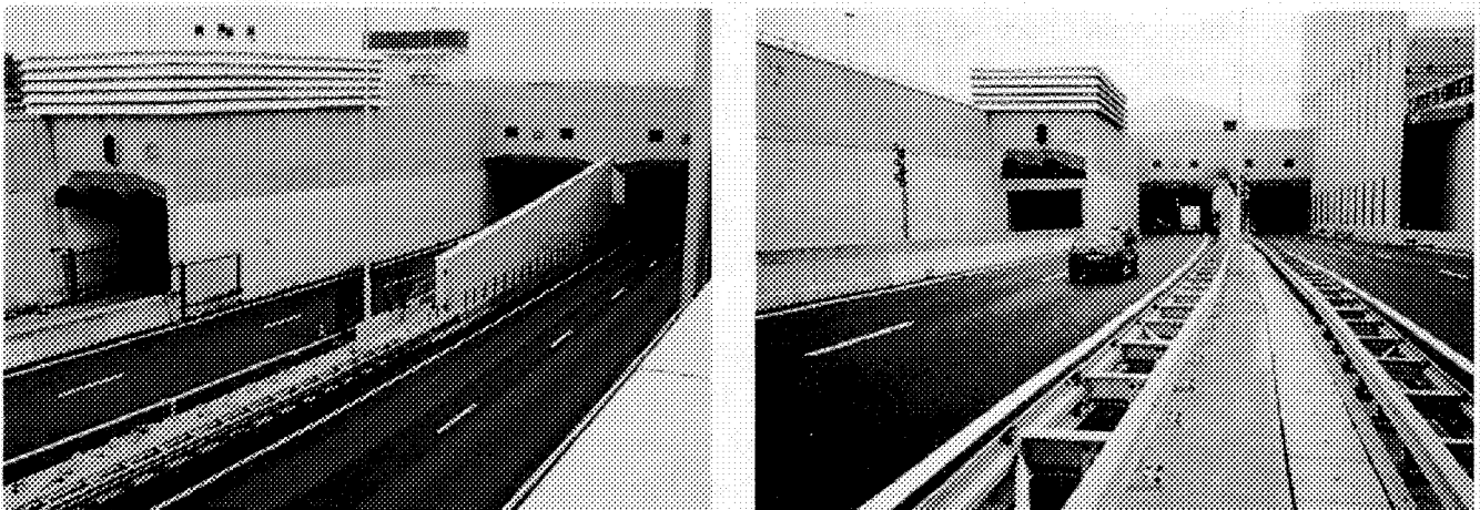
Fig. 4 Van links naar rechts de C-, D- en E-buis van de Beneluxtunnel, gezien vanaf de Zuidoever. (De proeven vonden plaats in de D-buis. Deze figuur sluit aan bij Fig. 6.)
