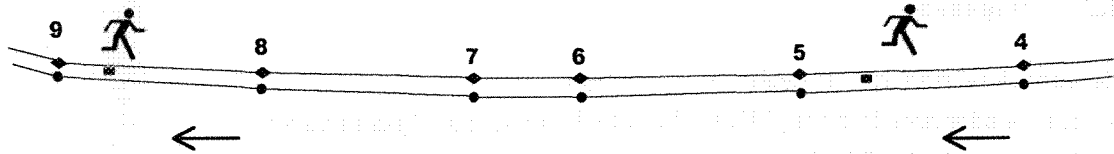
Fig. 9 Deelnemers komen aanrijden volgens de pijl, stoppen op aanwijzing van TNO tussen deur 8 en 9 (links) of tussen deur 4 en 5 (rechts) en moeten zich te voet in veiligheid brengen. Het beste is teruglopen naar een vluchtdeur (8 of 4). Doorlopen naar de dichtstbijzijnde vluchtdeur (9 of 5) is niet goed omdat de deelnemer dan langs de "ramp" moet.
