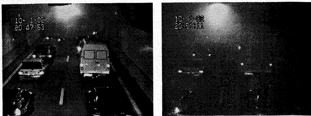
Fig. 16 De voorste auto's bij proef 6 verdwijnen geleidelijk in de rook maar de bestuurders blijven rustig zitten. (Gestreefd werd naar een langzame rook-afvoer in de rijrichting; bij deze proef was er te veel "tegenventilatie".)
