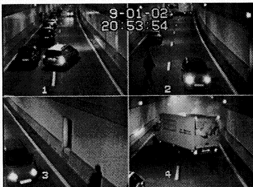
Fig. 15 Alternatieve evacuatie bij proef 4: terugrijden over de vrije rechterbaan. Inmiddels zijn er voetgangers op de baan.
