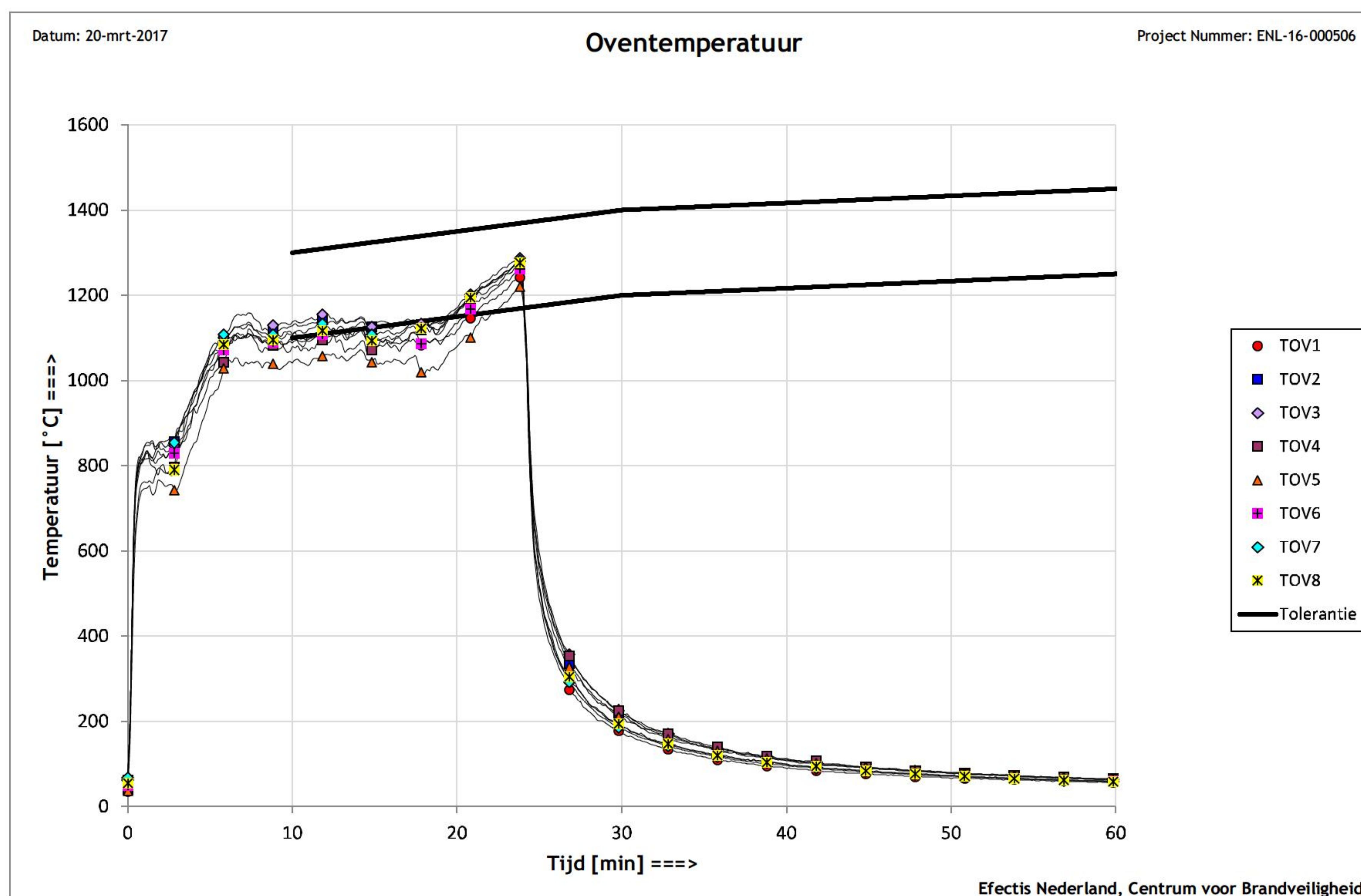
Figuur 1: Oventemperatuur
