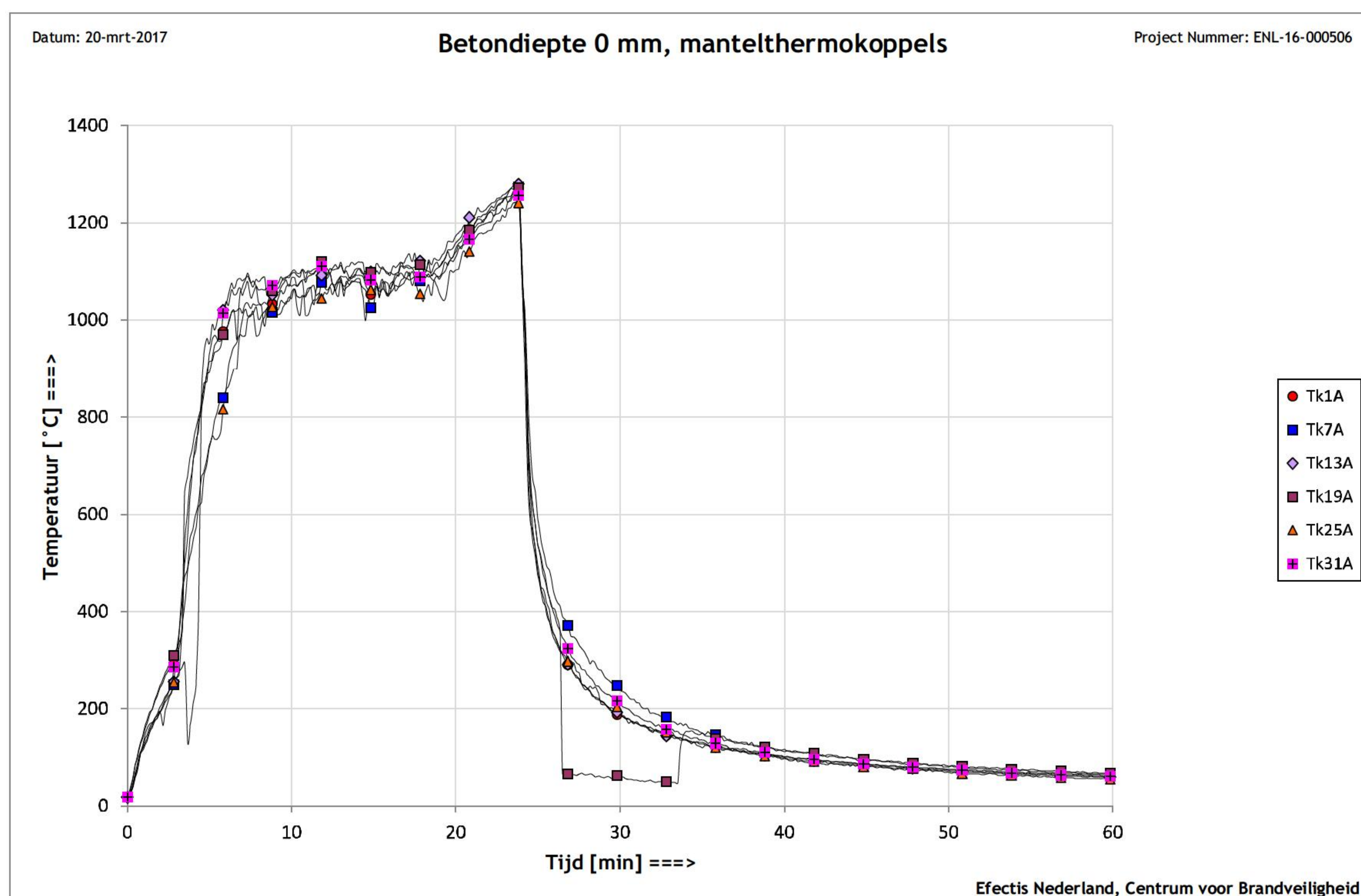
Figuur 5: Temperaturen gemeten aan het betonoppervlak – mantelthermokoppels
