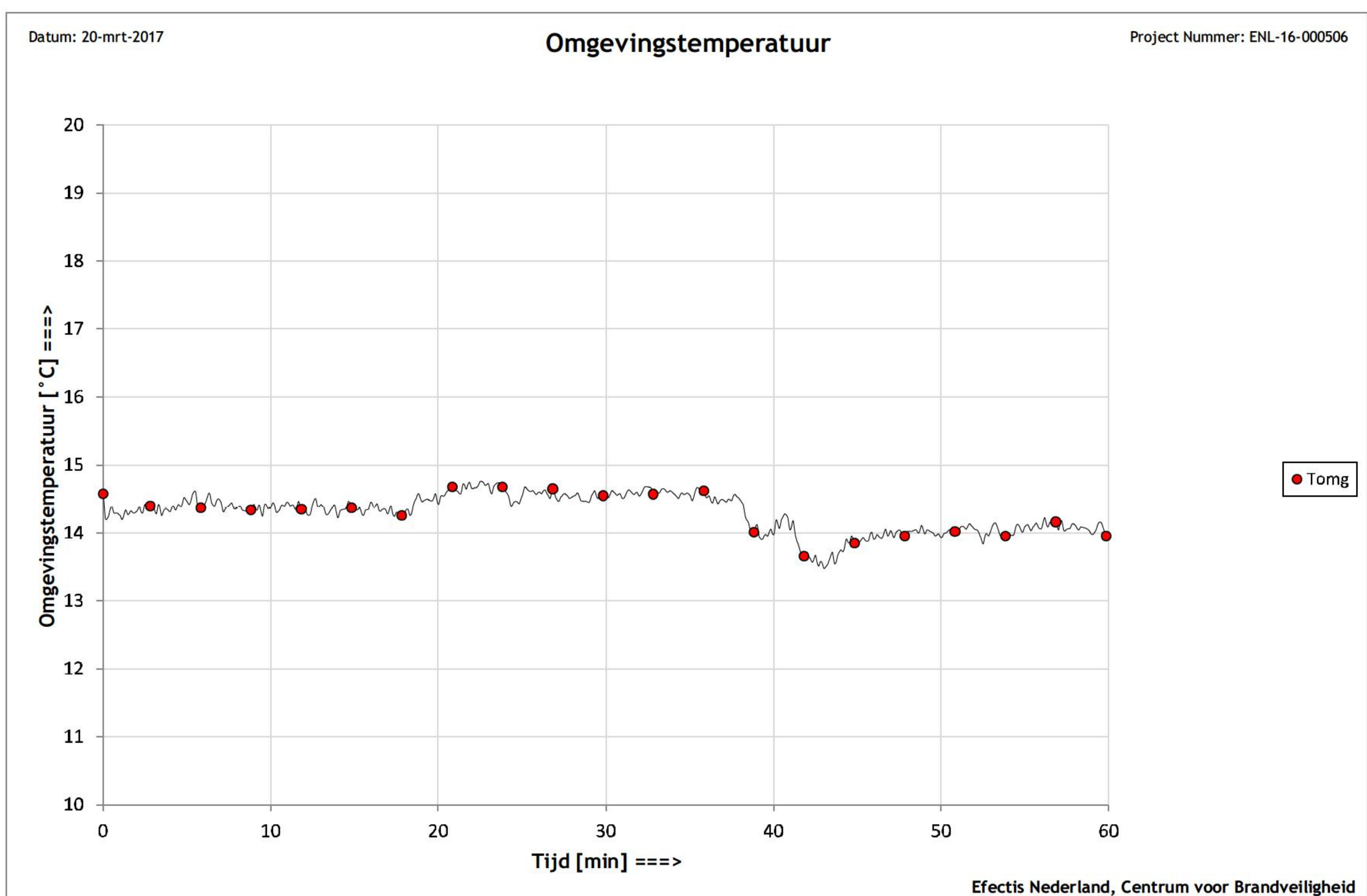
Figuur 3: Omgevingstemperatuur
