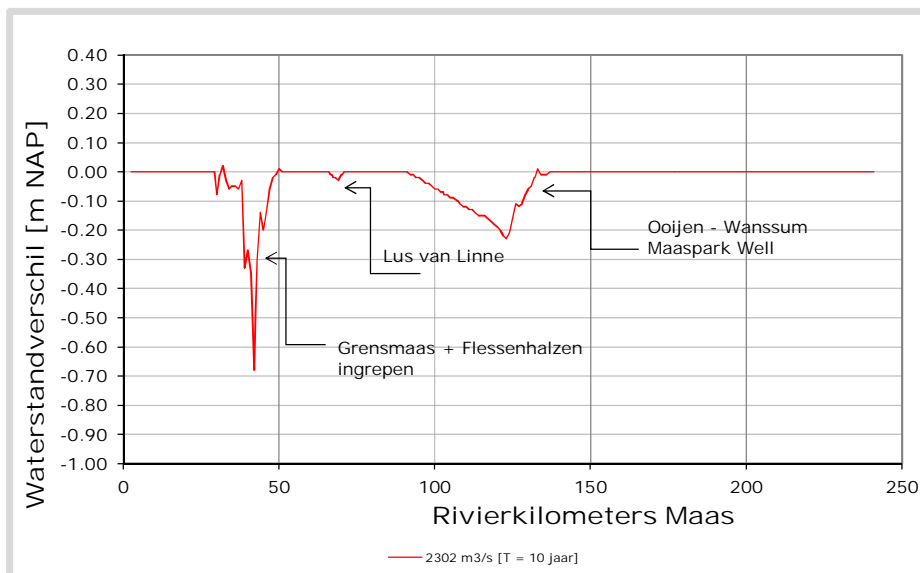
Figuur 1: verwachte extra waterstand effecten komende periode 2018/2019 t/m 2019/2020 van in uitvoering zijnde ingrepen die nog niet in de vigerende betrekingslijnen zijn verwerkt
