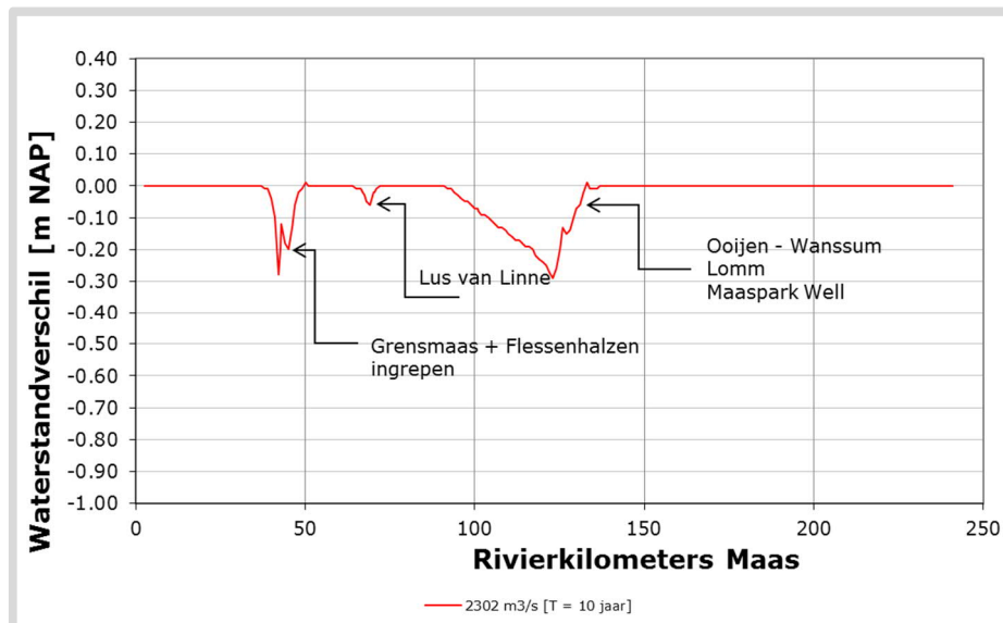
Figuur 1: verwachte extra waterstand effecten komende periode 2019/2020 t/m 2020/2021 van in uitvoering zijnde ingrepen die nog niet in de vigerende betrekkinglijnen zijn verwerkt
