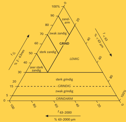
Figuur 15. RGD grinddriehoek
